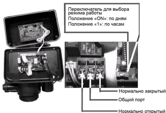
Рис.2. Настройка регенерации по дням или часам
