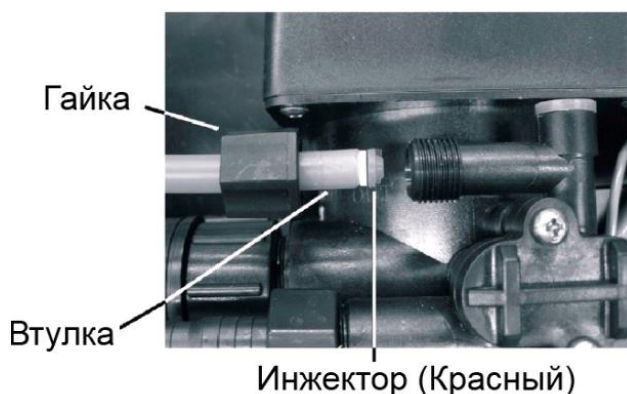
Рис.1. Подключение солевого бака
