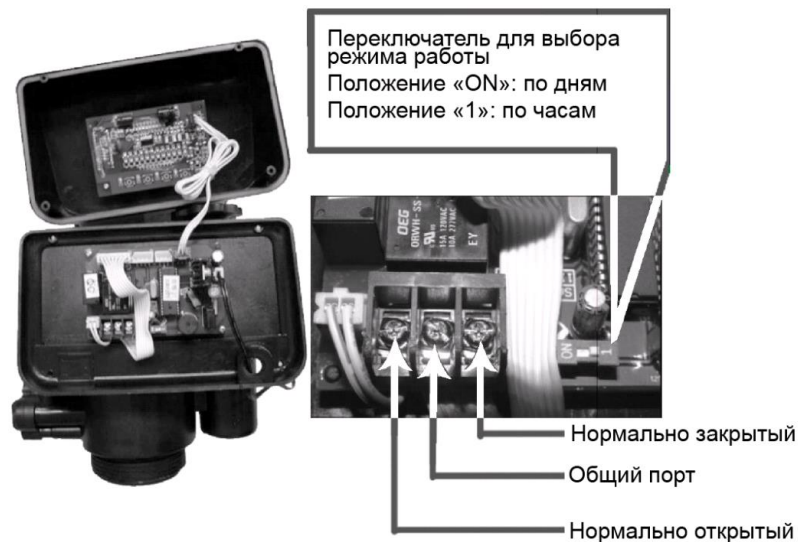
Рис.2. Настройка регенерации по дням или часам
