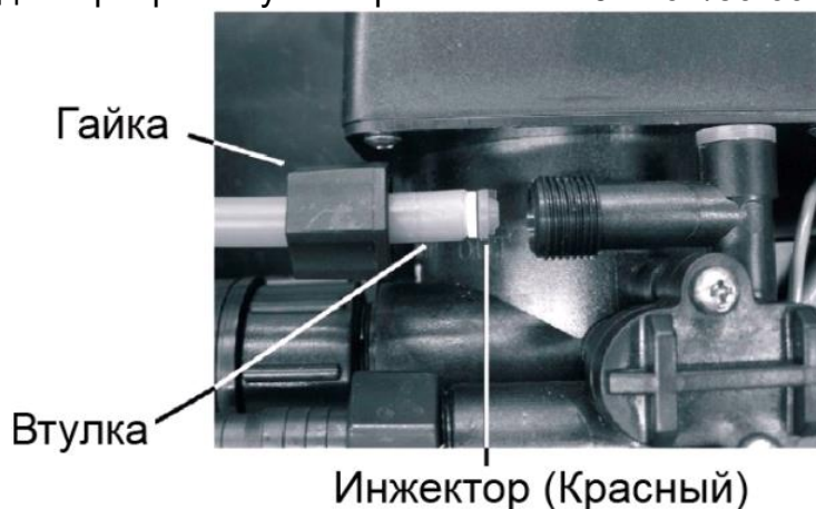
Рис.1. Подключение солевого бака к управляющему клапану
