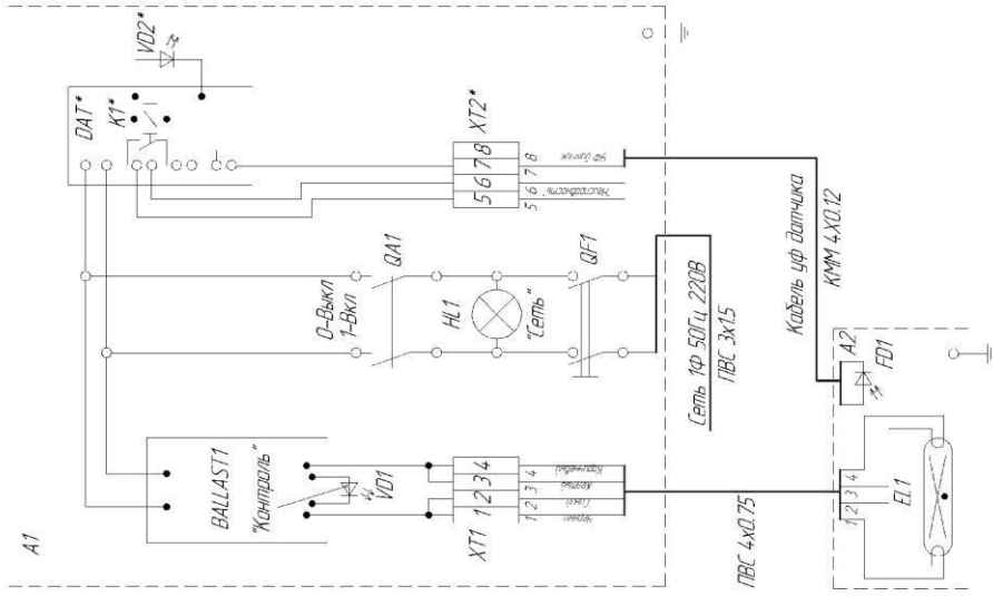
Вариант 1 с УФ Датчиком
