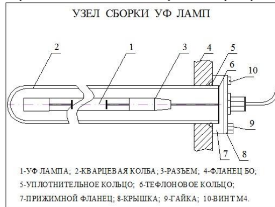
Рис. 2 Узел сборки ламп
