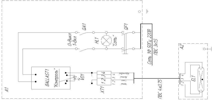
Вариант 2 без Уф Датчика
